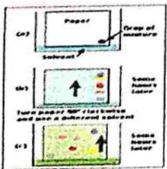
1. కాగితం క్రొమటోగ్రఫీ
